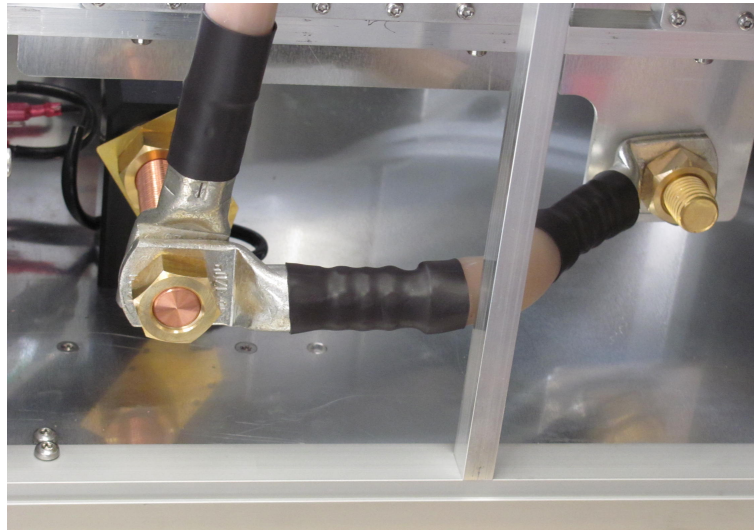
Abb. 6. Sicht auf die Kurzschlussbrücke „BNB 8656 L1/L2 short“ in „HV+“ Pfad. Fig. 6. View of the shorting bridge "BNB 8656 L1/L2 short" in "HV+" path.
