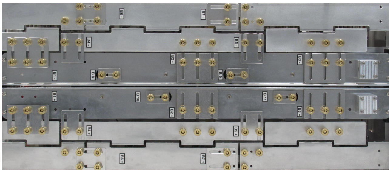
Abb. 11. Konfigurationsbeispiel für 2 x ( R_{int} = 10 \text{ m}\Omega ). Brücken B1, B6 sind eingesetzt.
