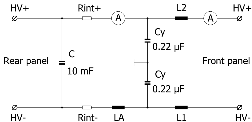
Abb. 3. Schaltplan nach Lastenheft VW 80300:2021-02. Fig. 3 Circuit diagram according to specification VW 80300:2021-02.
